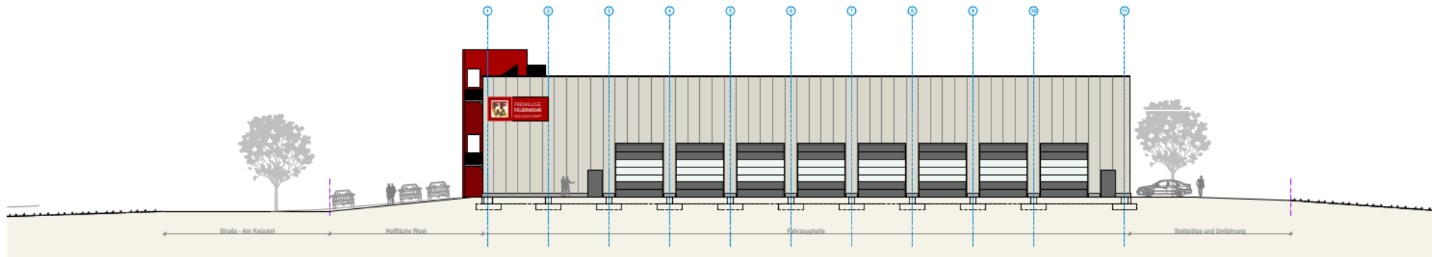
ANSICHT SÜD · ALARMAUSFAHRT
