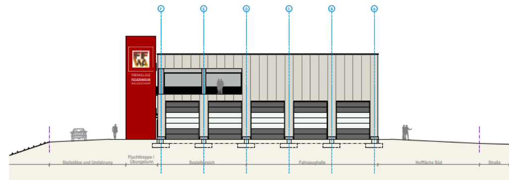
ANSICHT WEST · ALARMAUSFAHRT · AM KNÜCKEL
